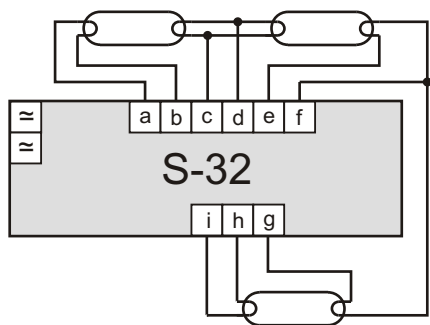
Statecznik: konfiguracja-S32
