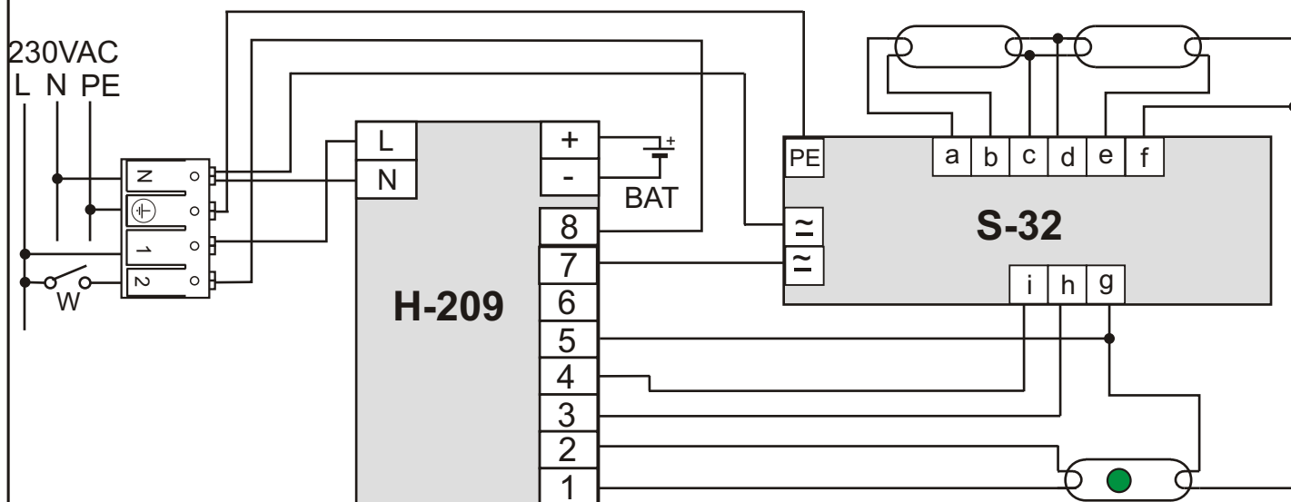
Statecznik: konfiguracja-S32
