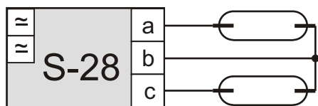
Statecznik: konfiguracja-S28
