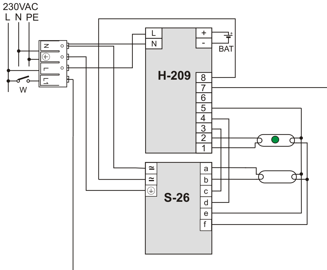
Statecznik: konfiguracja-S26
