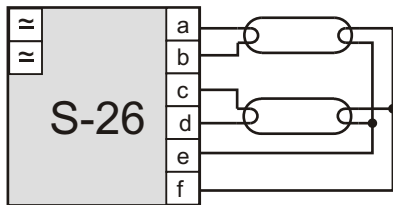
Statecznik: konfiguracja-S26
