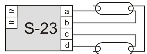
Statecznik-konfiguracja-S-23
