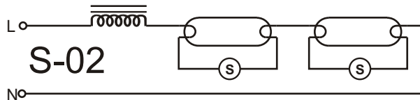
Statecznik: konfiguracja S-02
