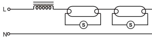
konfiguracja statecznika S-02
