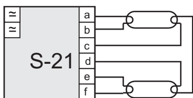
Statecznik-konfiguracja S21
